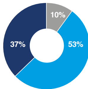
Oman
