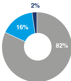
Kuwait
